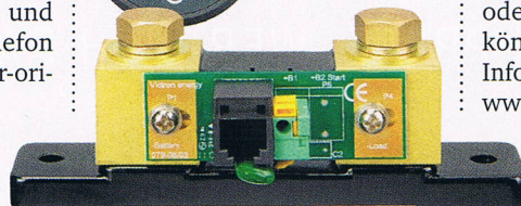
Batteriewächter der BMV-700-Serie mit Display und Shunt.
